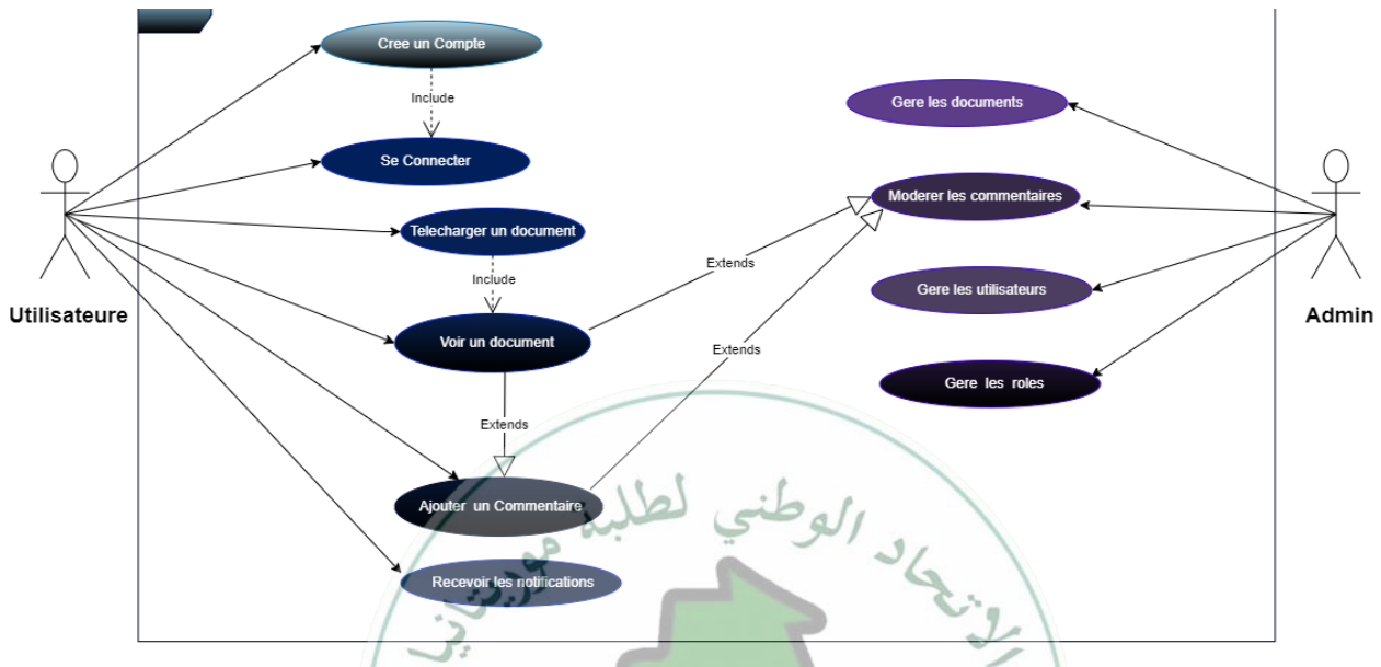
FIGURE 2 DIAGRAMME DE CAS D'UTILISATION
